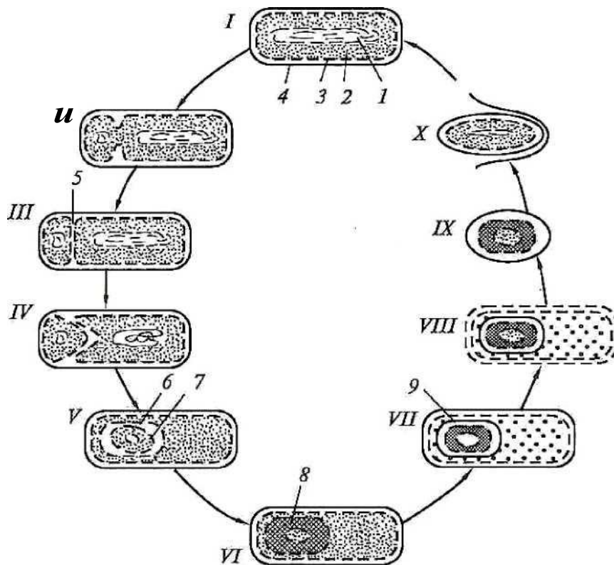
Рис. 7. Формирование эндоспоры:
