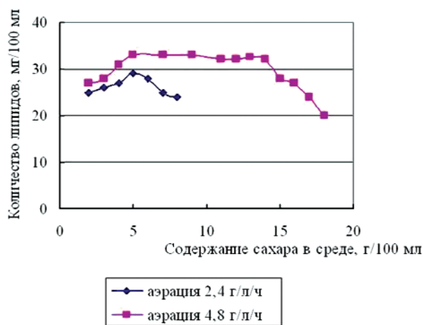
Рис. 1. Влияние содержания сахара в среде на синтез липидов дрожжами Rhodotorula gracilis SK-4 при разной скорости аэрации
