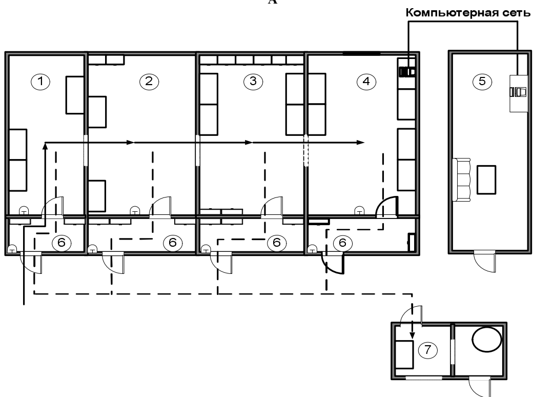
Рис.1. Рекомендуемые схемы размещения помещений (рабочих зон) лаборатории, использующей МАНК с электрофоретической и (или) гибридационно-ферментативной детекцией продуктов амплификации (А и Б).
