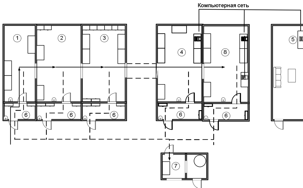
Рис.3. Рекомендуемая схема размещения помещений (рабочих зон) лаборатории, использующей МАНК с комплексной детекцией продуктов амплификации (электрофоретической, гибридно-ферментативной (ГИФА), гибридно-флуоресцентной), а также их последующего секвенирования или проведения анализа на ДНК-чипах.
