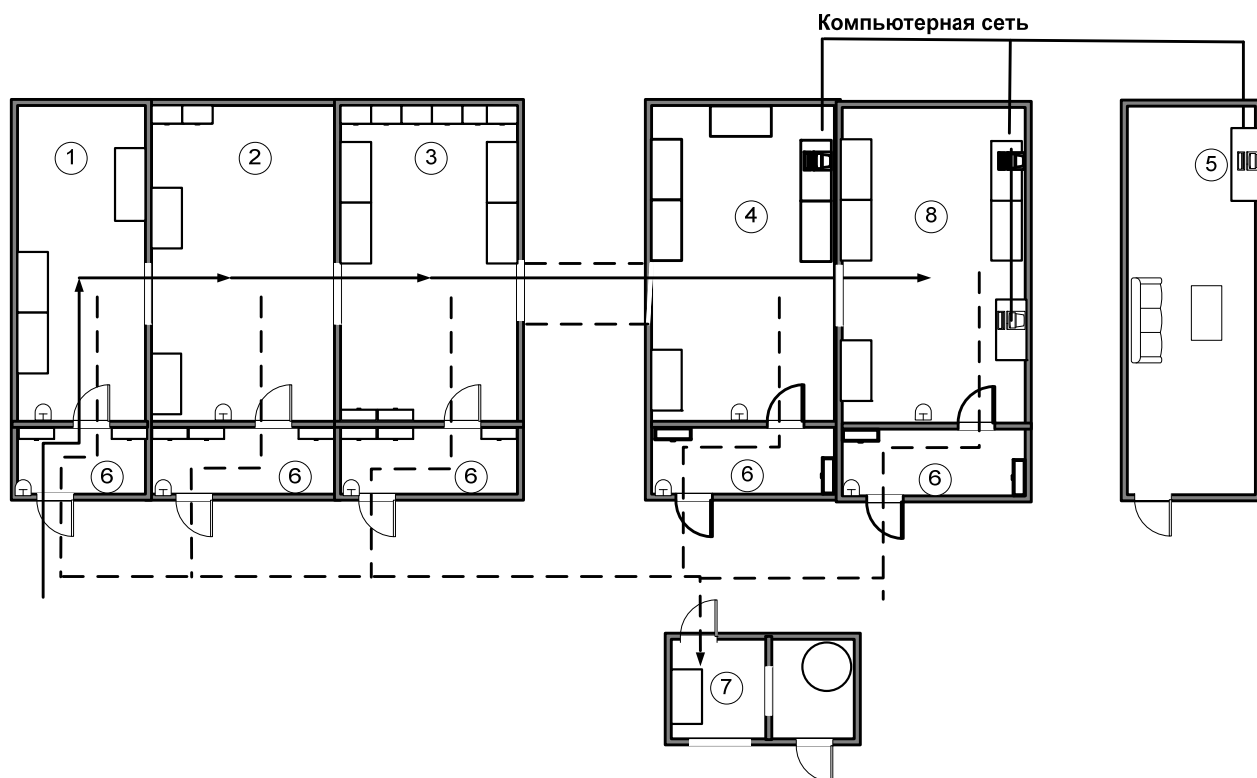
Рис.3. Рекомендуемая схема размещения помещений (рабочих зон) лаборатории, использующей МАНК с комплексной детекцией продуктов амплификации (электрофоретической, гибридационно-ферментативной (ГИФА), гибридационно – флуоресцентной), а также их последующего секвенирования или проведения анализа на ДНК-чипах.
