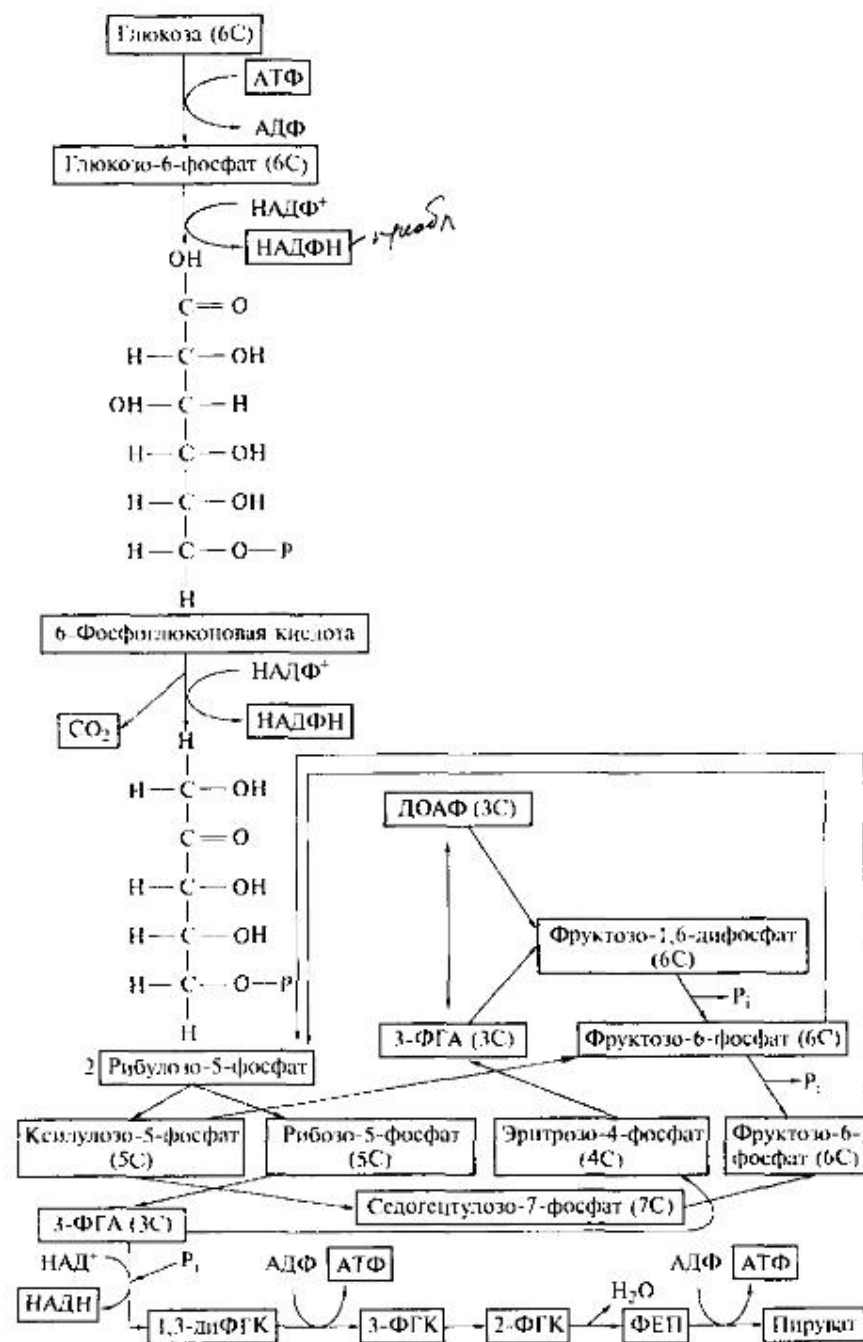
Рис. 82. Пентозофосфатный путь
