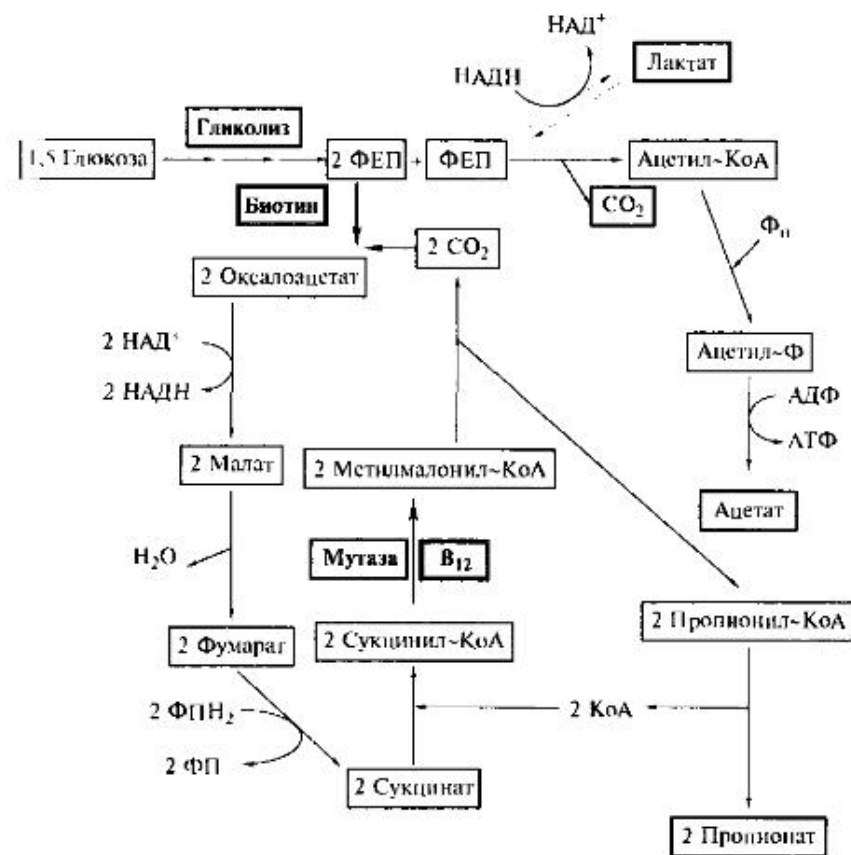
Рис. 92. Пропионовокислое брожение
