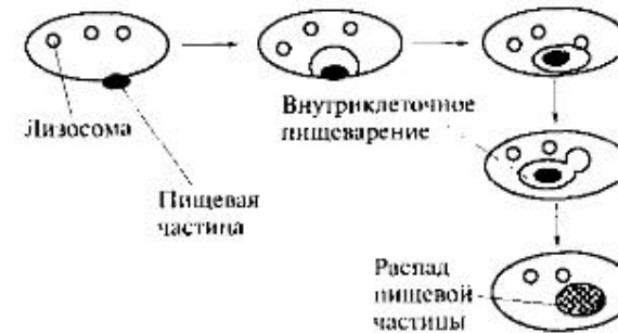
Рис. 74. Эндоцитоз
