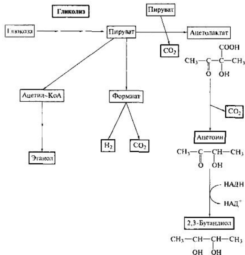
Рис. 94. Бутандиоловое брожение
