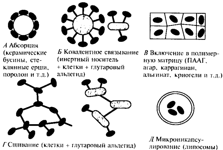
Рис. 173. Виды иммобилизации:
