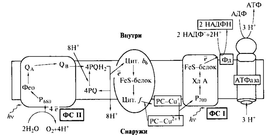
Рис. 131. Транспорт электронов при фотосинтезе (обозначения см. на рис. 130)
