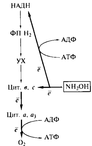
Рис. 124. Схема ЭТЦ (с обратным переносом электронов) у нитрификаторов I фазы
