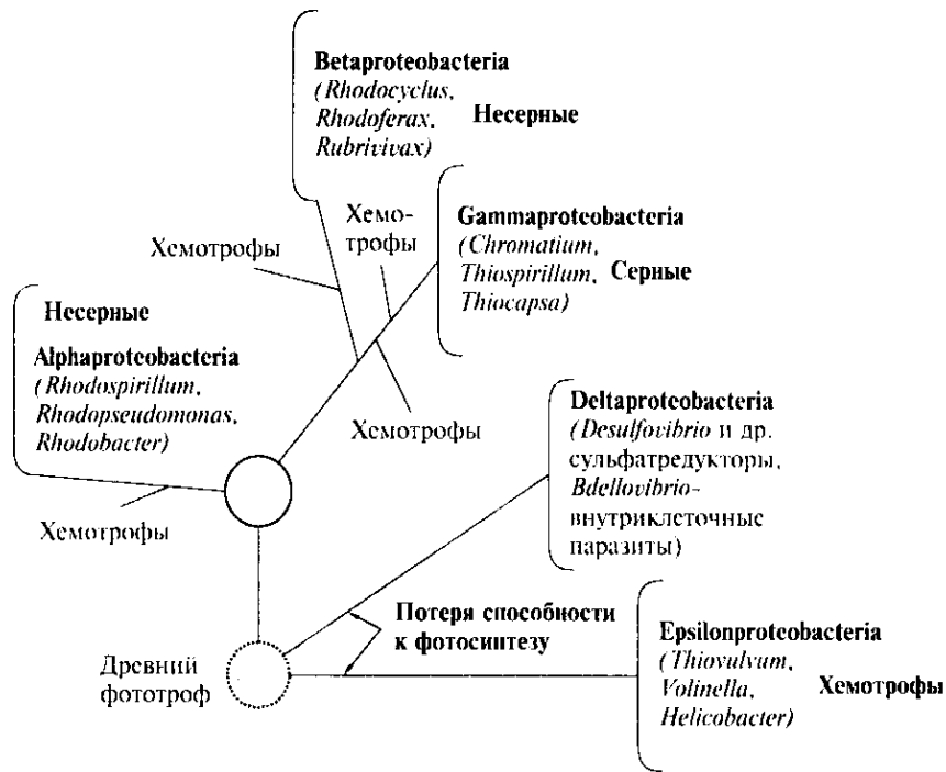
Рис. 135. Место пурпурных бактерий в филуме Proteobacteria
