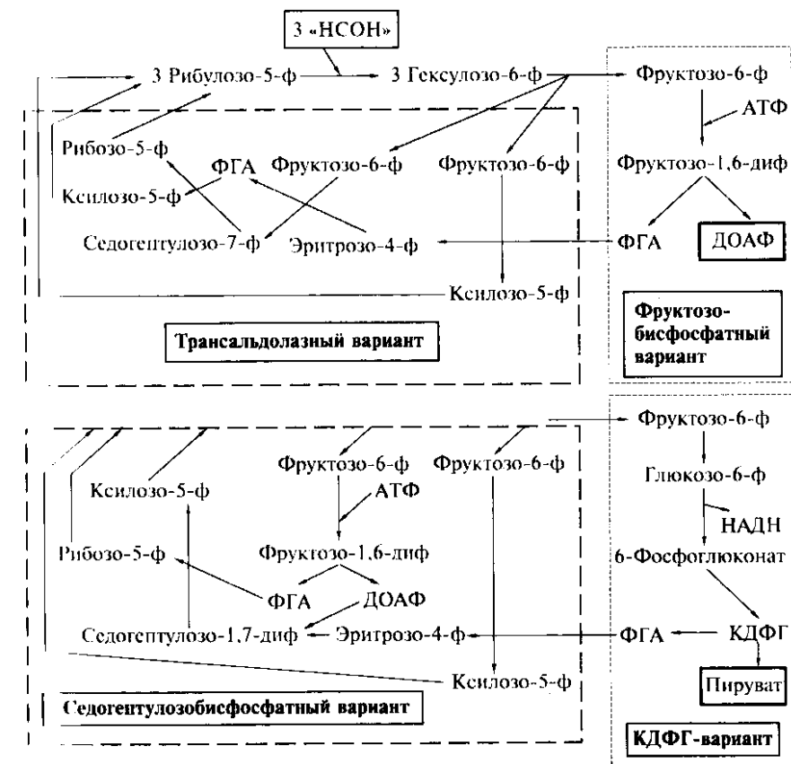
Рис. 114. Рибулозобисфосфатный цикл (РМФ-цикл) (ф — фосфат)
