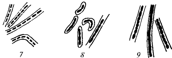
Рис. 10. Различные формы нитчатых бактерий:
