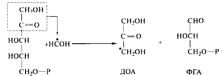
Рис. 123. Первая реакция в ДОА-цикле (ДОА — диоксиацетон)
