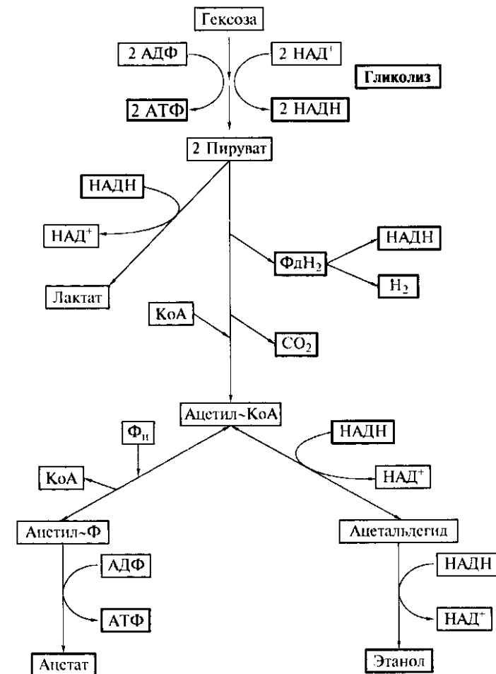
Рис. 87. Спиртовое брожение некоторых энтеробактерий и кластридий
