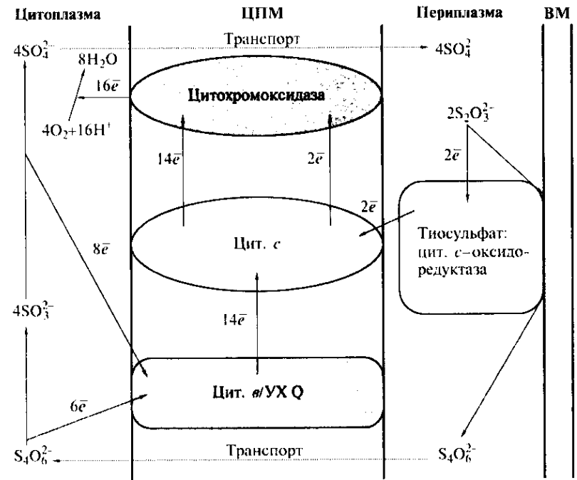
Рис. 128. Пространственная организация ЭТЦ некоторых тиобацилл
