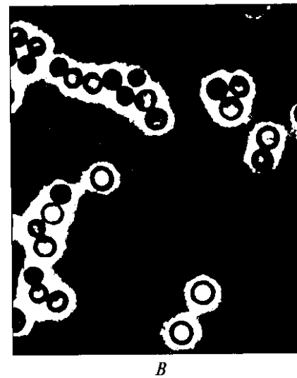
Рис. 60. Различные формы клеток миксобактерий, образующих плодовые тела:
