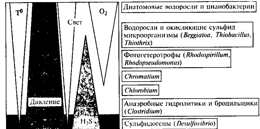
Рис. 165. Модель водной экосистемы с градиентами основных факторов и распределением групп микроорганизмов
