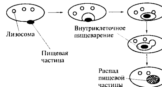
Рис. 74. Эндоцитоз
