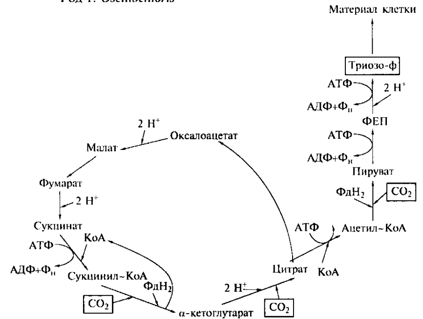
Рис. 136. Цикл Арнона у зеленых серных бактерий
