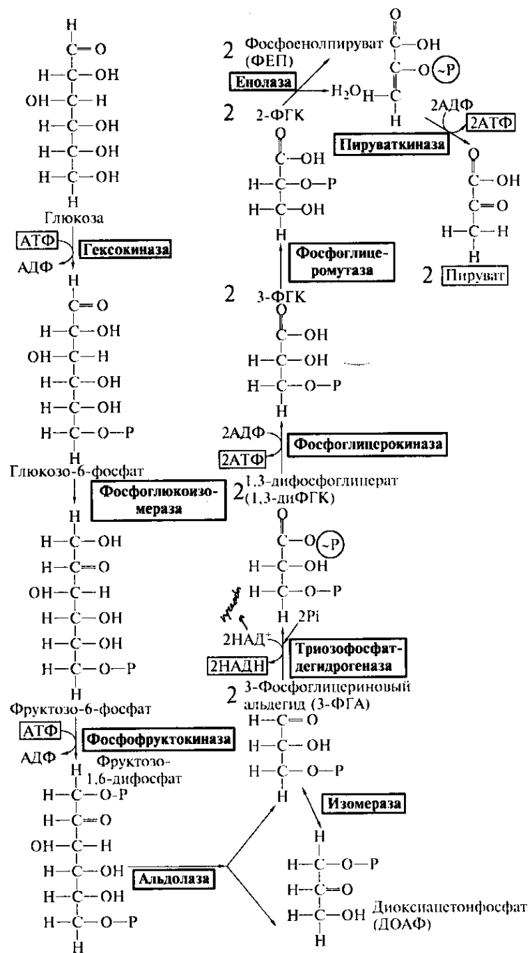
Рис. 81. Гликолиз
