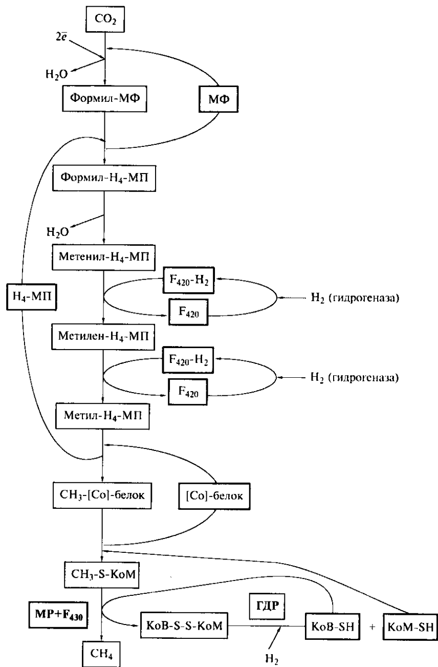
Рис. 104. Процесс образования метана на \text{H}_2/\text{CO}_2 (МФ — метанофурил; \text{H}_4 -МП — тетрагидрометаноптерин, МР — метилредуктаза; ГДР — гетеродисульфидредуктаза)
