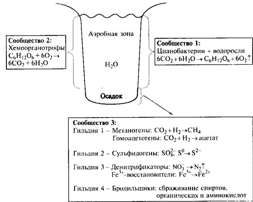
Рис. 164. Модель сообществ микроорганизмов непроточного озера
