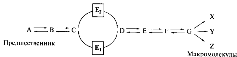
Рис. 144. Простейшая схема регуляции амфиболических путей (активация фермента E_2 приводит к сдвигу реакций в сторону биосинтеза, E_1 — в сторону расщепления)
