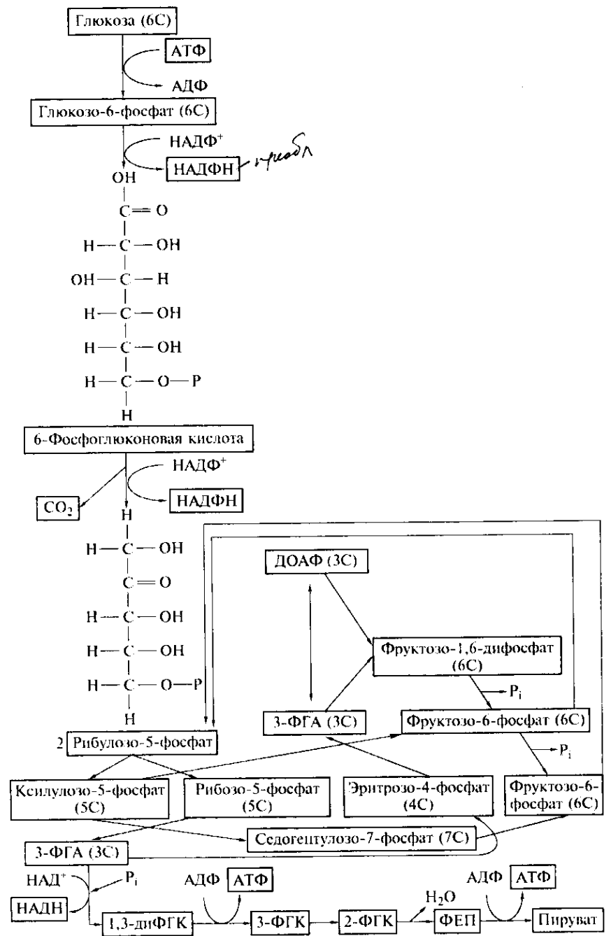
Рис. 82. Пентозофосфатный путь
