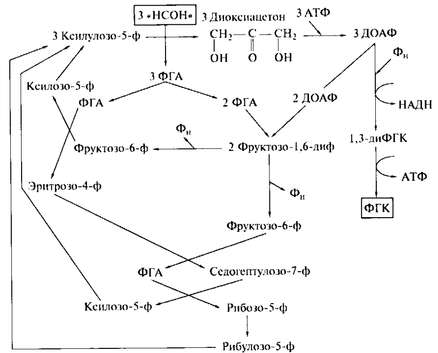
Рис. 116. Диоксиацетоновый цикл фиксации формальдегида
