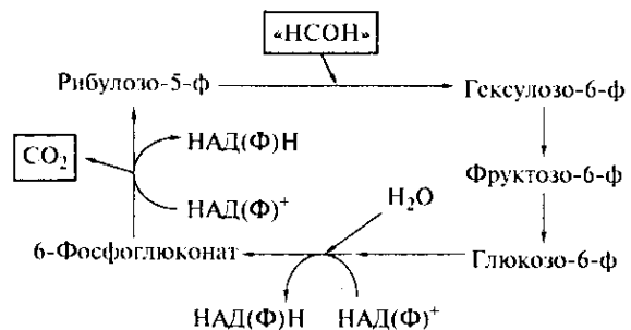
Рис. 118. Диссимиляционный цикл окисления формальдегида
