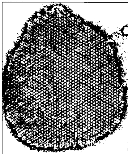
Рис. 45. Правильный слой белковых гексагональных структур на внешней стороне клеточной стенки спироилл. Подобные S-слои найдены и у многих грамположительных бактерий, однако они легко теряют регулярную структуру при приготовлении препаратов (негативное контрастирование, увел. 200 000 x )
