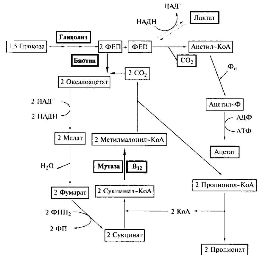
Рис. 92. Пропионовокислое брожение
