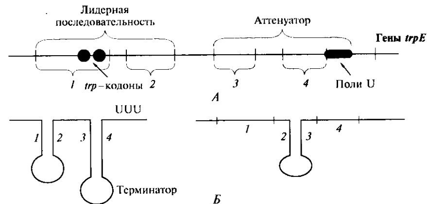
Рис. 158. Расположение групп нуклеотидов в ДНК (А) и разные варианты образования «шпилек» (Б) при аттенуации (1—4 — сегменты ДНК)
