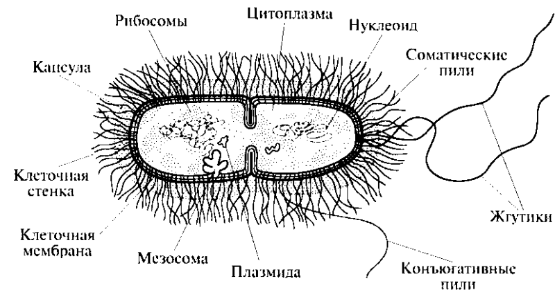
Рис. 14. Схема делящейся бактериальной клетки
