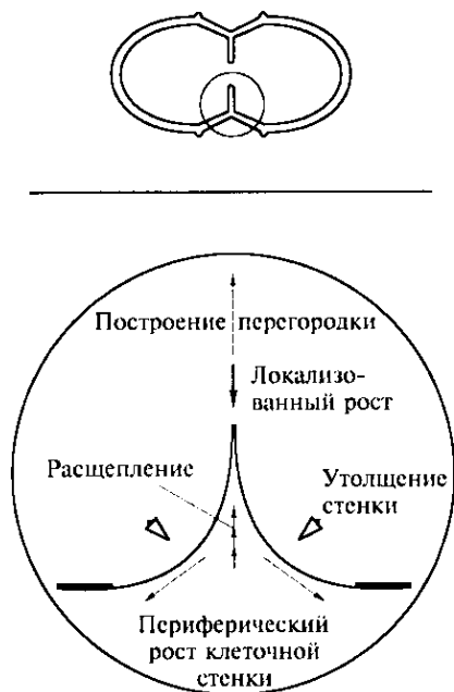
Рис. 149. Схема нарастания клеточной стенки (перегородки или перетяжки) при делении бактериальной клетки. Часть делящегося кока, обведенная окружностью, показана детально на нижней части рисунка. Черная стрелка обозначает место нарастания нового материала переднего конца септы. Группа из трех небольших стрелок показывает места действия гидролаза муреина, которые разделяют вновь образованный материал. В результате новый материал выталкивается наружу, увеличивая поверхности двух дочерних клеток. Две белые стрелки указывают места утолщения, три пунктирные стрелки показывают направления увеличения периферических стенок и нарастания центральной перегородки. Старый слой пептидогликана показан черным
