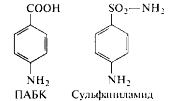
Рис. 69. Структурные аналоги
