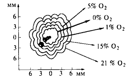
Рис. 160. Распределение кислорода в комочке хорошо аэрируемой почвы
